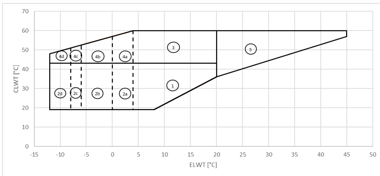
Slika10 - EWWS_VZ_SS
