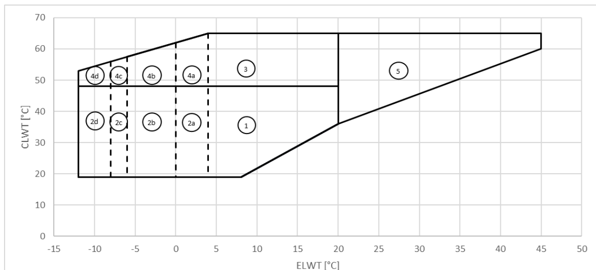
Slika6 - EWWD-VZ-XS/PS
