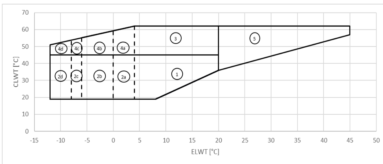
Slika11 - EWWS_VZ_XS/PS
