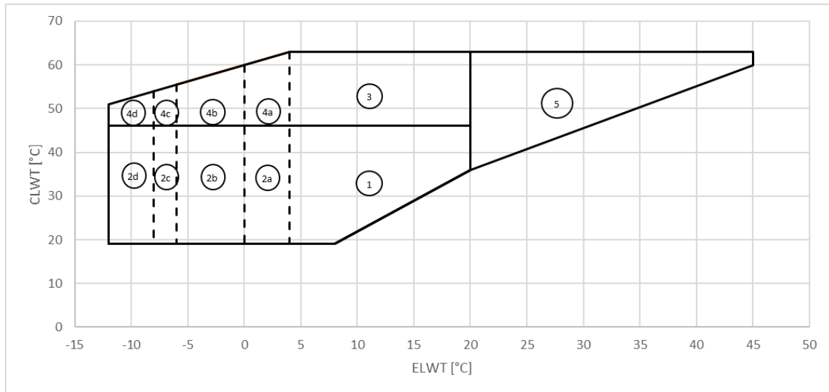
Slika5 - EWWD_VZ_SS
