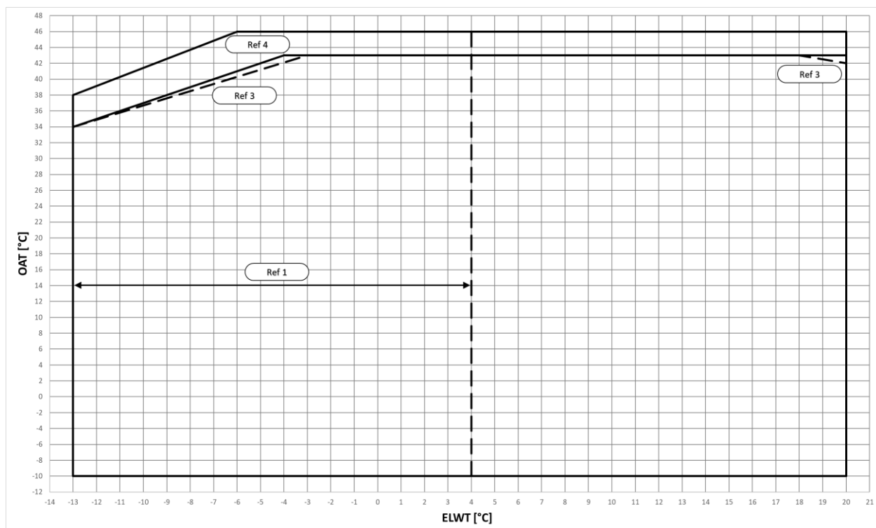
Sl. 2 – Radne granice EWYTx5B-X moda hlađenja
