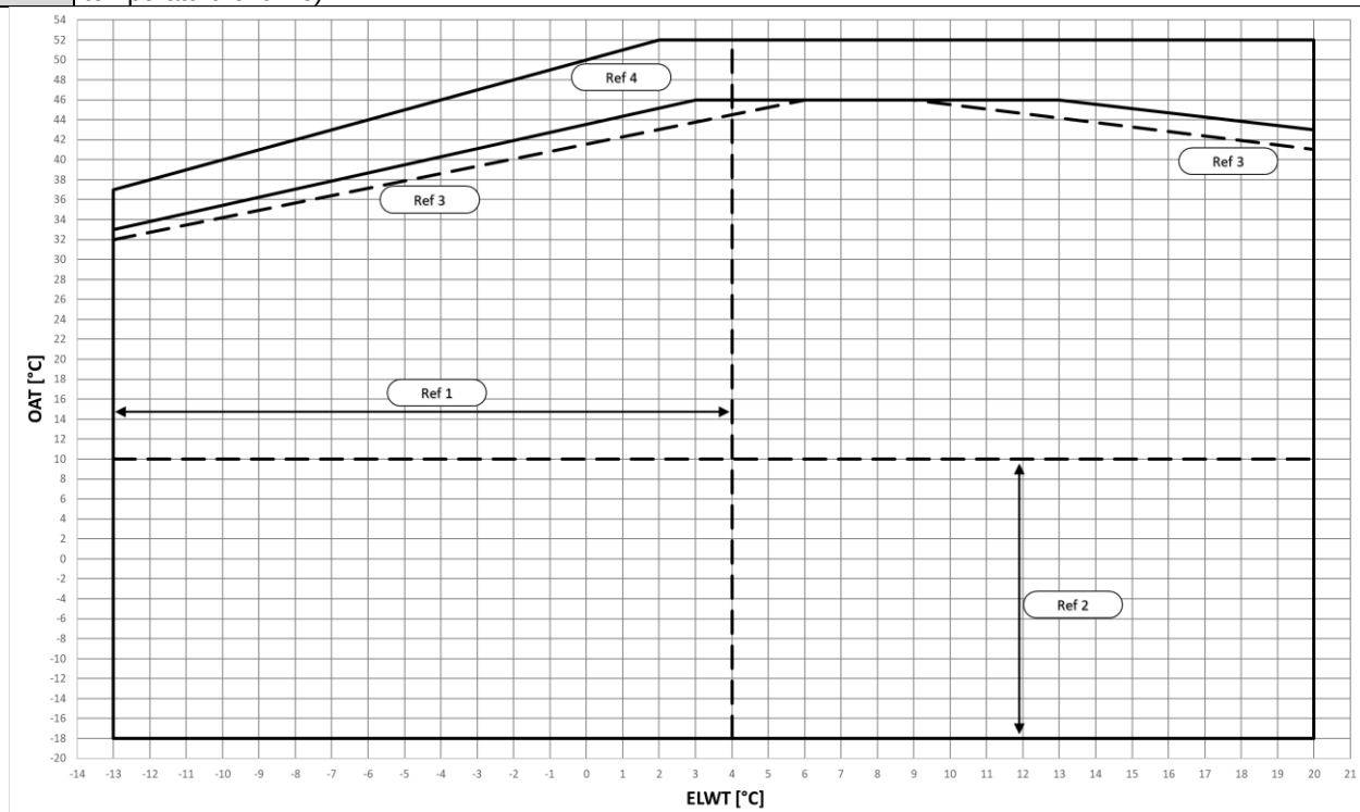
Sl. 3 – Radne granice EWYTx0B-S načina hlađenja
