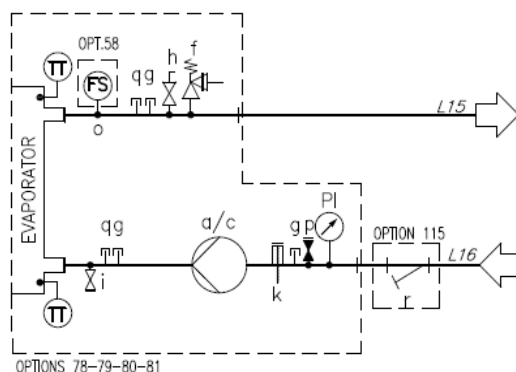
Sl. 15 – Hidraulički dijagram za jednu pumpu / dvostruku pumpu (EWYTx5B) (opt. 78-79) (maks. radni tlak 6 bara)
