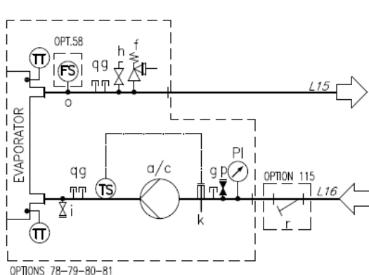
Sl. 17 – Hidraulički dijagram za dvostruku pumpu (EWYTx5B) (opcija 80-81/136-137) (maks. radni tlak 6 bara)
