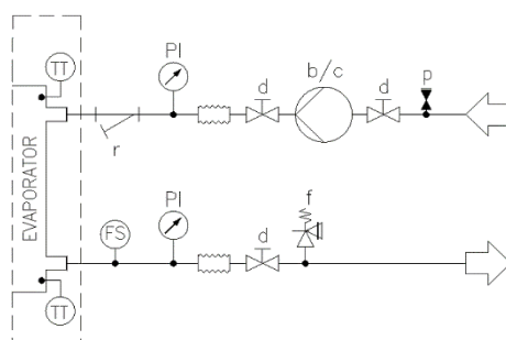
Sl. 14 – Hidraulički dijagram bez pumpi na brodu (maks. radni tlak 20 bar)
