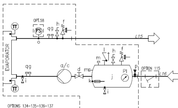
Sl. 16 – Hidraulički dijagram za jednu pumpu / dvostruku pumpu s spremnikom (EWYTx5B) (opt. 134-135) (maks. radni tlak 6 bara)
