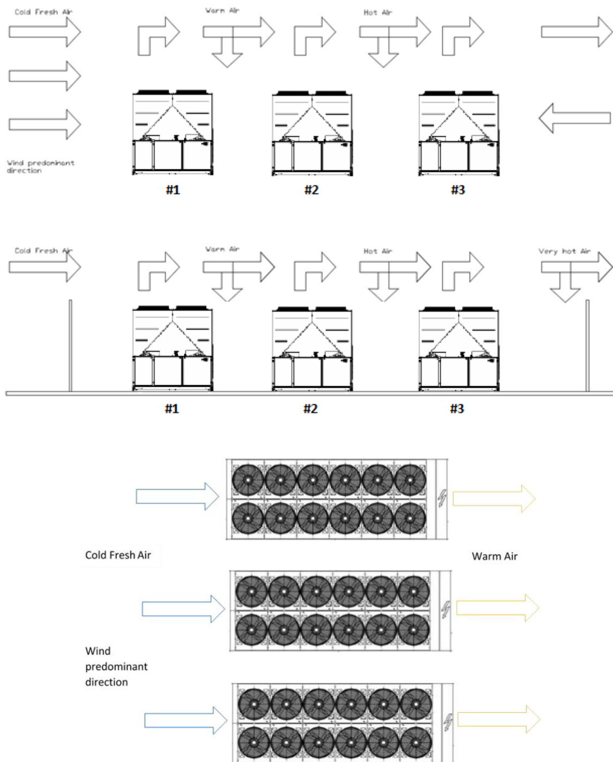
Sl. 12 – Instalacija višestruke jedinice (način hlađenja)
