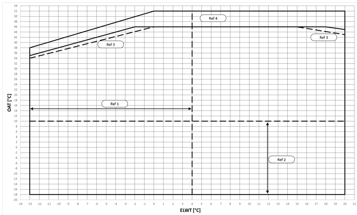
Sl. 4 – Radne granice EWYTx0B-X moda hlađenja
