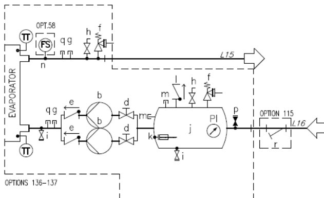
Sl. 17 – Hidraulički dijagram za dvostruku pumpu (EWYTx5B) (opcija 80-81/136-137) (maks. radni tlak 6 bara)
