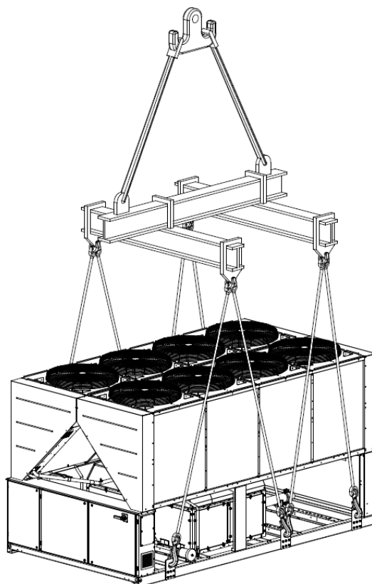
Jedinica s 6 točki podizanja
