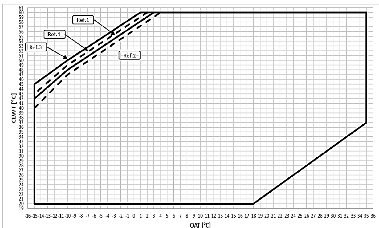
SI. 8 – EWYT ~B-X – OP.204 Ograničenja rada načina grijanja
