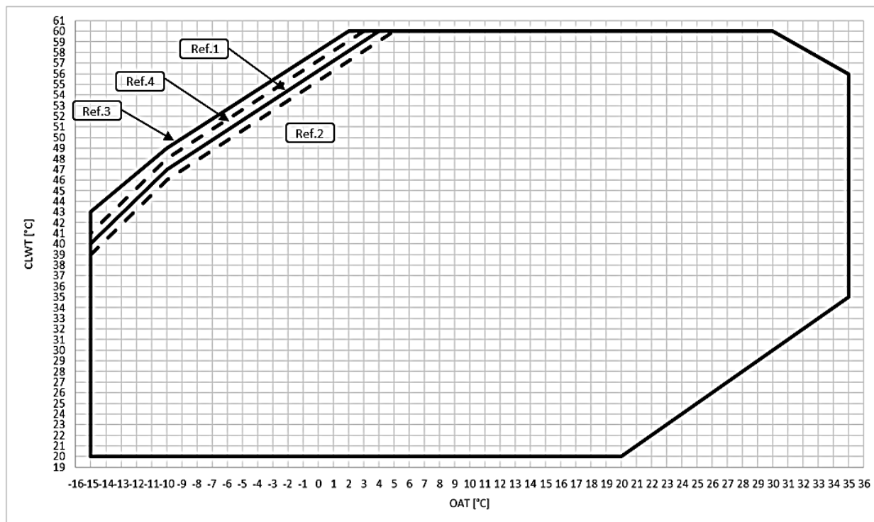
Sl. 7 – EWYT-B-S – OP.204 Ograničenje rada načina grijanja
