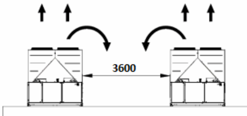
Sl. 11 – Minimalni zahtjevi za prostor
