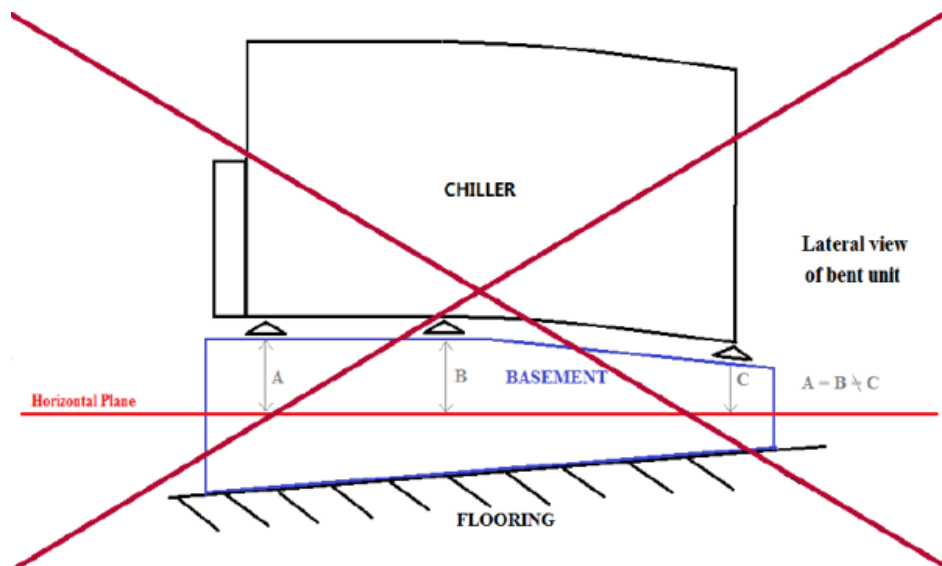
Sl. 10 – Izravnavanje jedinice
