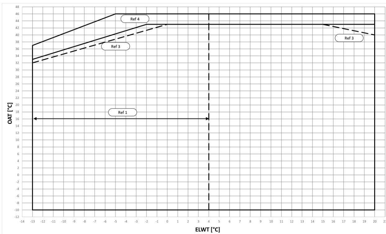
Sl. 1 – Radne granice EWYTx5B-S načina hlađenja
