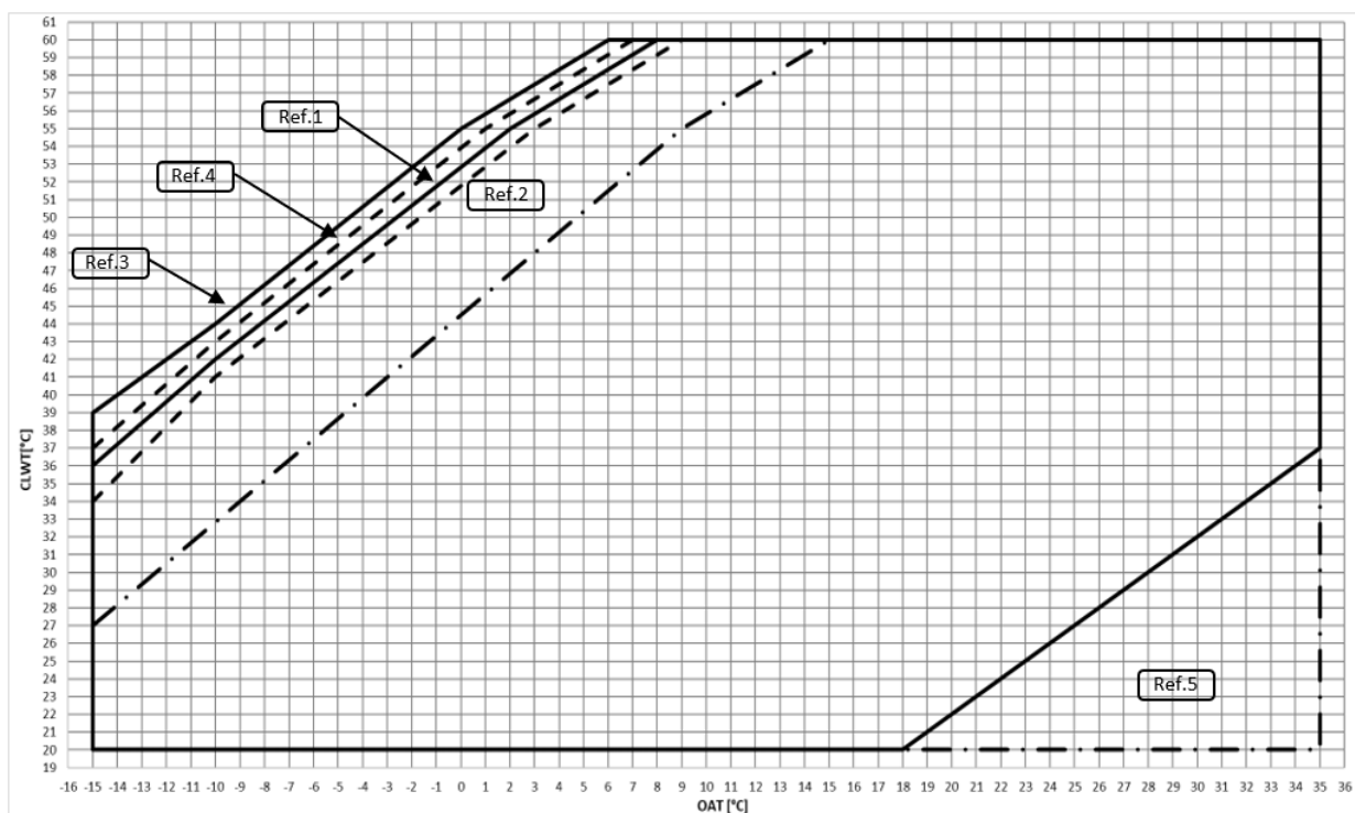
Sl. 6 – Radne granice EWYT ~ B-X načina grijanja
