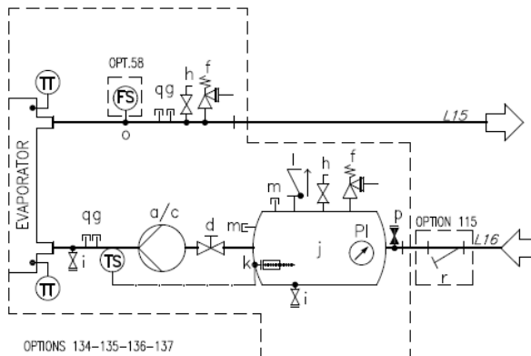
Sl. 17 – Hidraulički dijagram za dvostruku pumpu (EWYTx5B) (opcija 80-81/136-137) (maks. radni tlak 6 bara)
