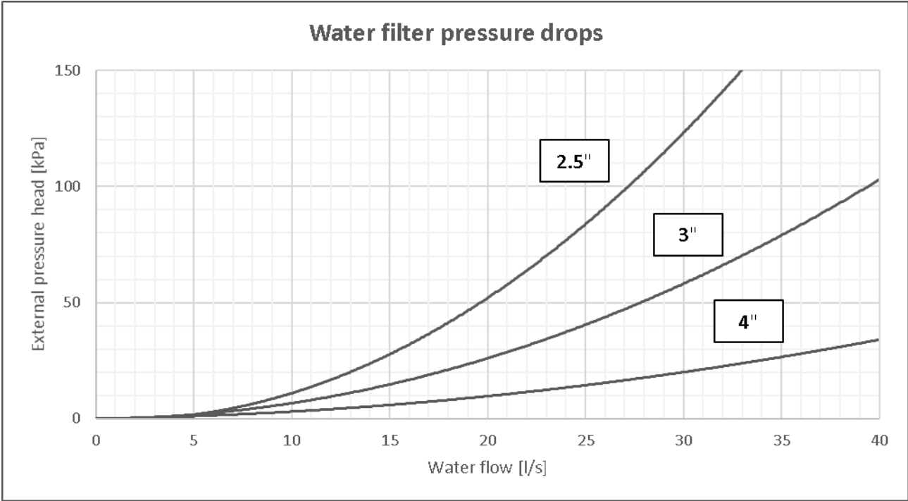
Sl. 13 – Pad tlaka filtra za vodu
