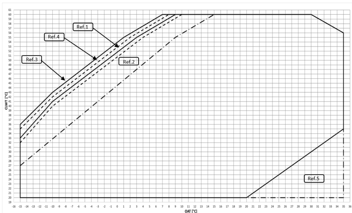
Sl. 5 – Radne granice EWYT ~ B-S načina grijanja
