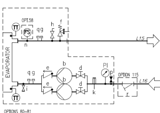
Sl. 17 – Hidraulički dijagram za dvostruku pumpu (EWYTx5B) (opcija 80-81/136-137) (maks. radni tlak 6 bara)
