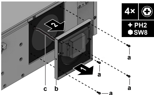
a Vijak b Prigušna zaklopka c Žica zaklopke
