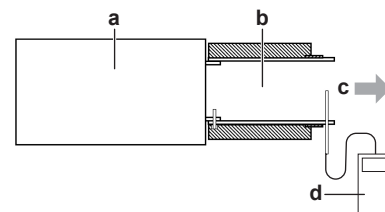
a SV jedinica b Kanal za izlaz zraka c Smjer strujanja zraka d Anemometar s vrućom žicom
