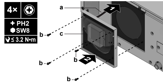
a Žica zaklopke b Vijak c Prigušna zaklopka
