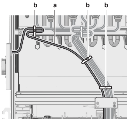
a Žica zaklopke b Kabelska vezica
