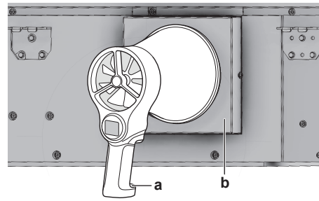
a Anemometar s lopaticama b Komplet za spajanje kanala (EKBSDCK)
