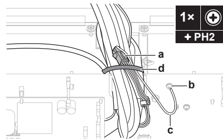
a Priključnica b Vijak žice za uzemljenje c Žica uzemljenja zaklopke d Kabelska vezica
