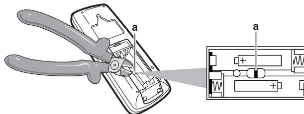
a Premosnik adrese
