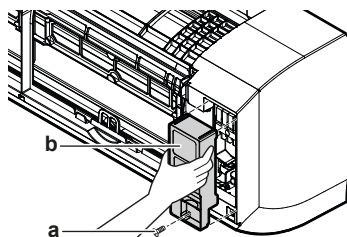
a Vijak pristupnog poklopca b Servisni poklopac
